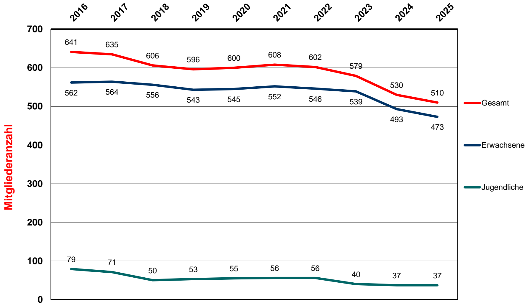
HBSV-Mitgliederstatistik 1
