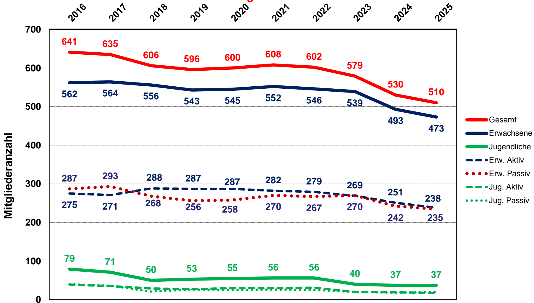
HBSV-Mitgliederstatistik 2
